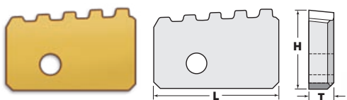
3/4" BUTTRESS SET 755P1E / 755P2E / 755P3E
