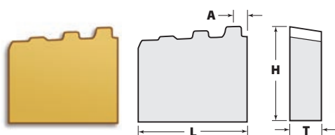
3/4" BUTTRESS SET 755P1E / 755P2E / 755P3E
