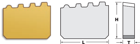
1" BUTTRESS SET 15P1E / 15P2E / 15P3E
