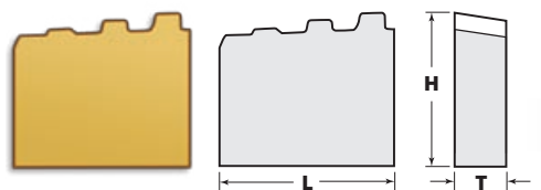
1" BUTTRESS SET 15P1E / 15P2E / 15P3E
