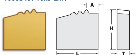
1003E (3T-10RD-EXT)
